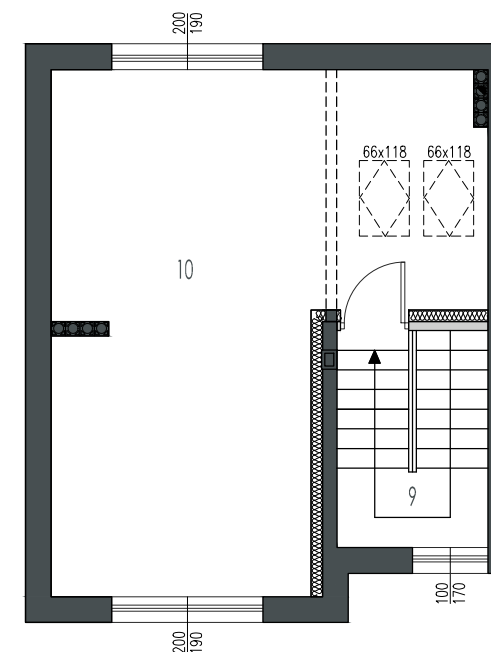
rzut strychu
