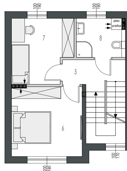
rzut piętra
