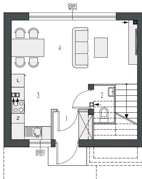
rzut parteru
