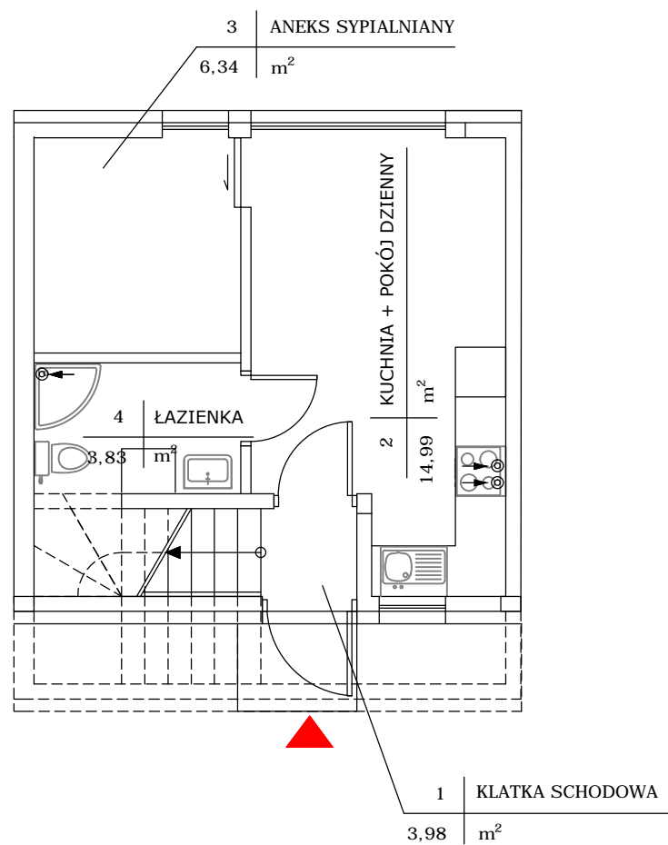
Kondygnacja parteru
