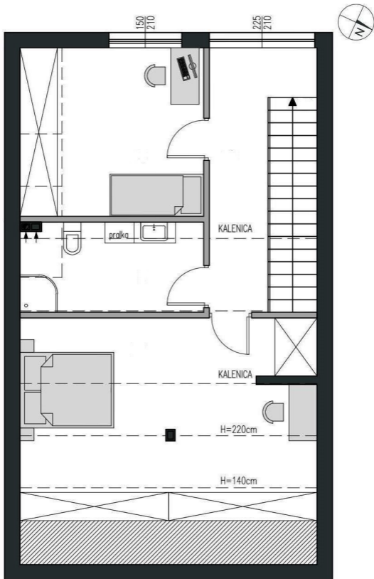
Przykładowa aranżacja strychu
